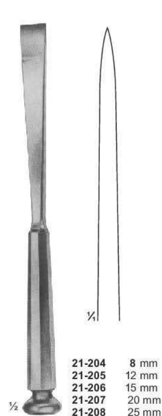
STILLE 21-204 - 208 Osteotomes 205 mm
